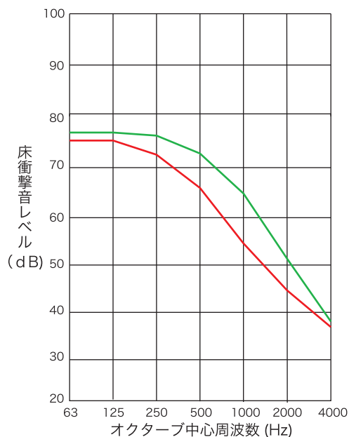
床衝撃音レベル（軽量）
