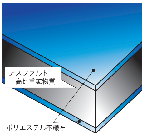
■ 断面構成図
