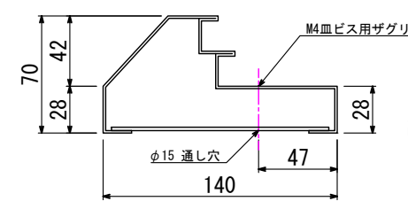
扉枠下部巻摺り枠ビス穴位置
