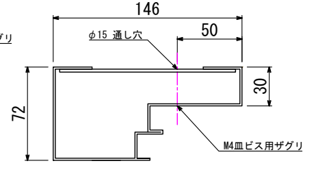
扉枠ビス穴位置
