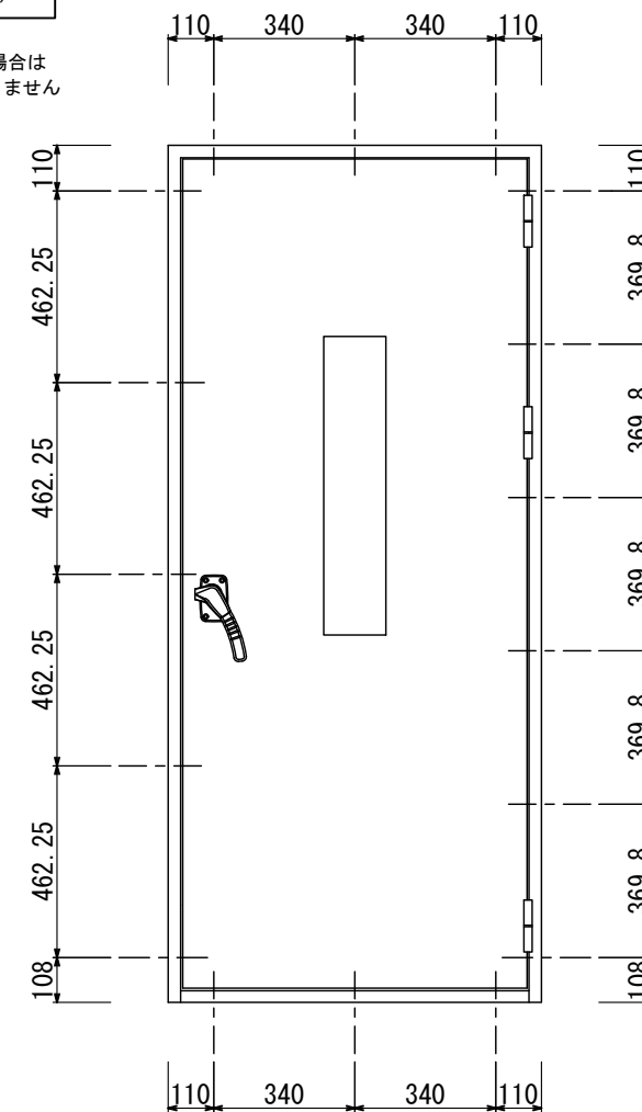
扉枠下部寄寄り枠ビス穴位置
