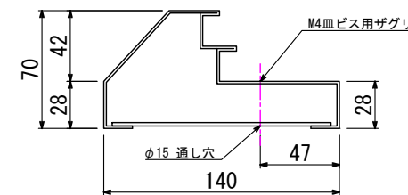
扉枠下部寄寄り枠ビス穴位置
