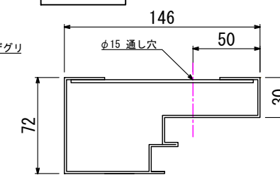
扉枠ビス穴位置
