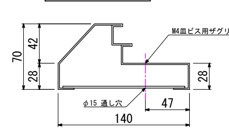
扉枠下部番摺り枠ビス穴位置
