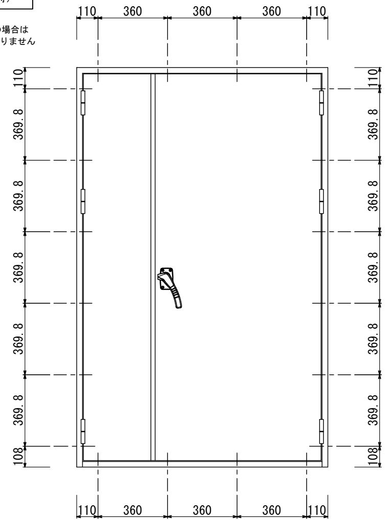
扉枠下部番摺り枠ビス穴位置
