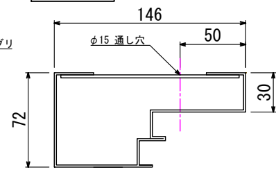
扉枠ビス穴位置
