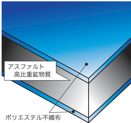
■ 断面構成図
